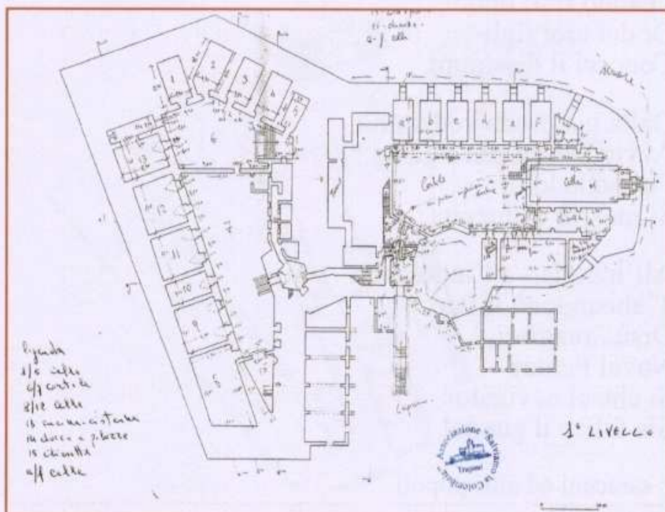
Planimetria del 1° livello (Arch. Ferranova)
